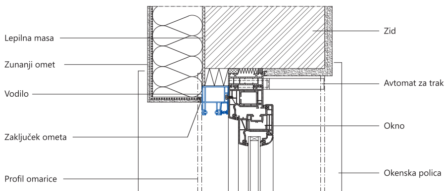
Vertikalni prerez Roltek KARO omarice 250
