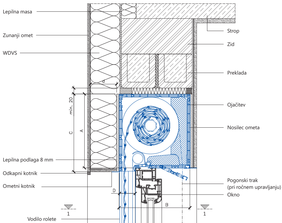
Horizontalni prerez Roltek KARO omarice 250
